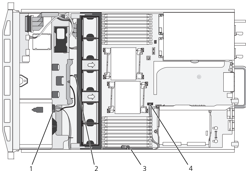
図 3-17. 光学ドライブケーブルの配線
