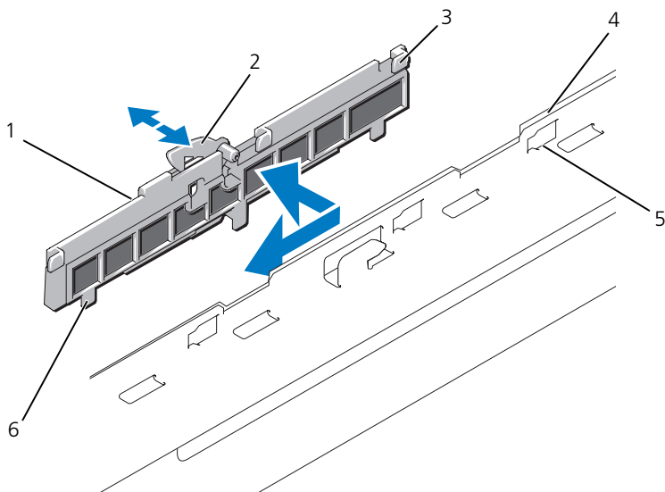
図 3-21. ケーブル保持ブラケットの取り外しと取り付け
