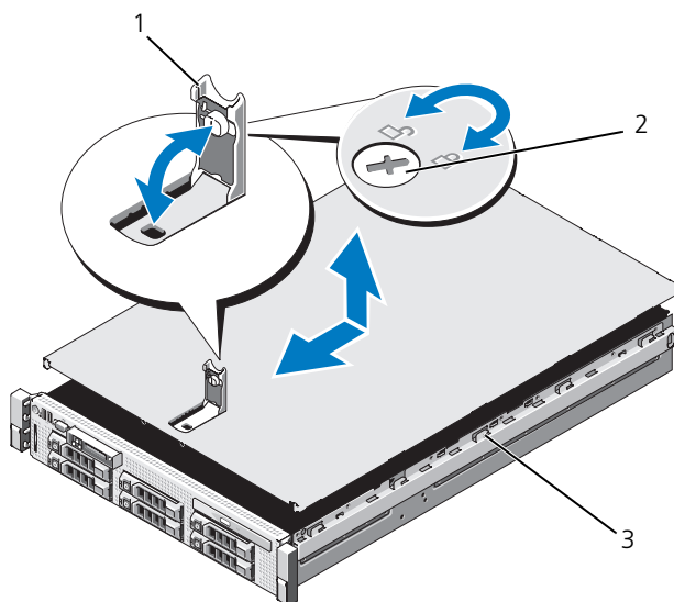
図 3-3. カバーの取り外しと取り付け
