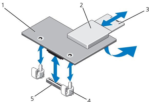
図 3-11. iDRAC6 Enterprise カードの取り外しと取り付け
