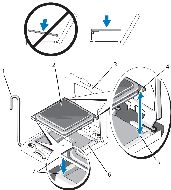
図 3-29. プロセッサの取り付けと取り外し
