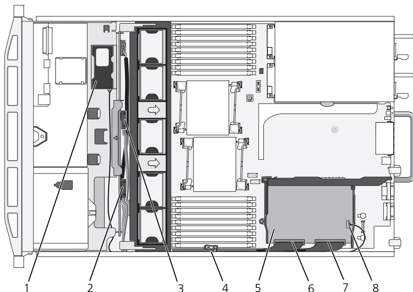
図 3-19. ストレージコントローラカードの配線
