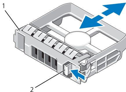
図 3-5. ハードディスクドライブダミーの取り外しと取り付け
