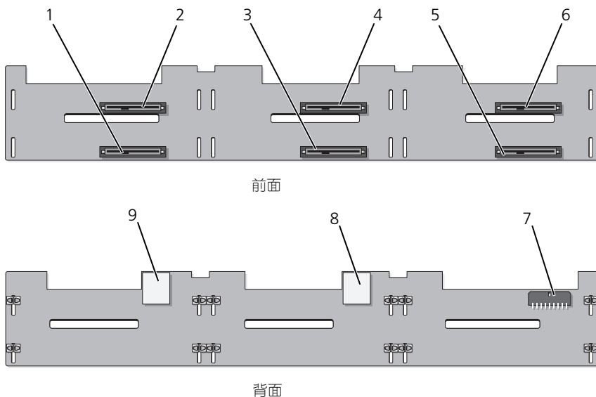
図 6-3. SAS バックプレーンボード (6 スロット)
