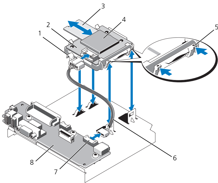
図 3-9. 内蔵 SD モジュールの取り外しと取り付け
