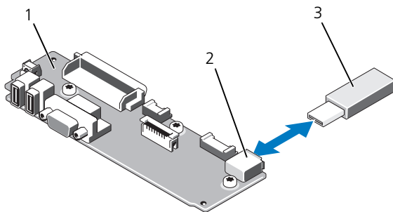
図 3-10. USB メモリキーの取り外しと取り付け
