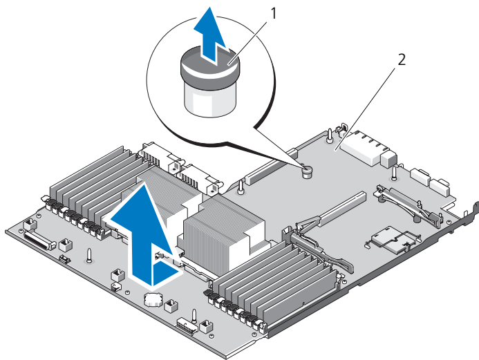
図 3-34. システム基板の取り外し
