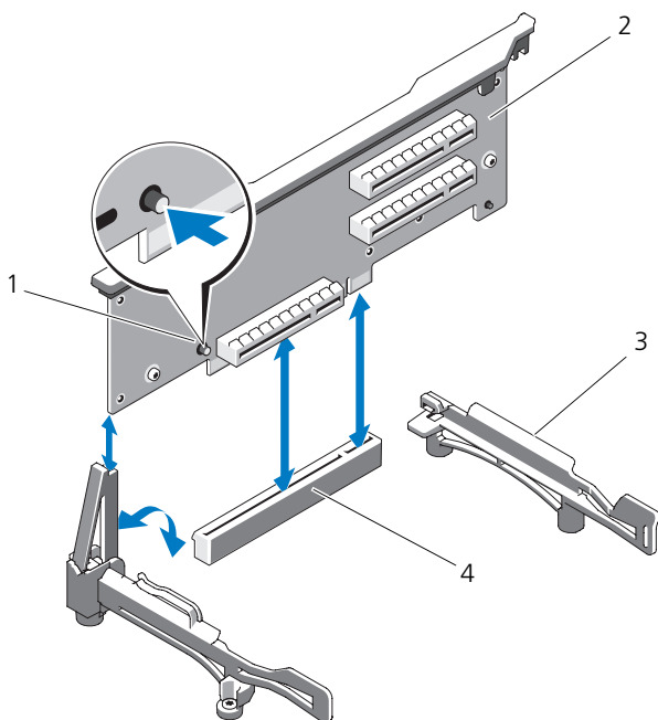
図 3-23. 拡張カードライザー 1 の取り外しと取り付け
