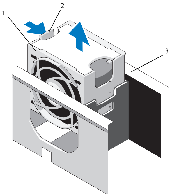
図 3-14. 冷却ファンの取り外しと取り付け
