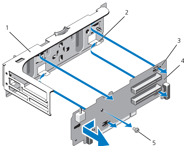
図 3-25. ライザー 2 ボードの取り外しと取り付け
