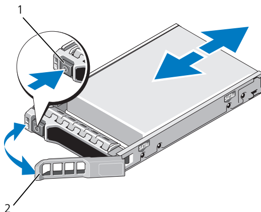
図 3-6. ホットスワップ対応ハードディスクドライブの取り付け
