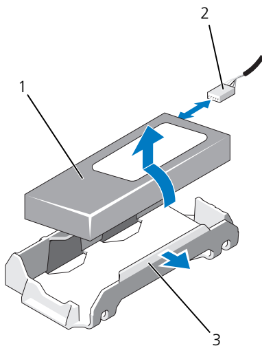
図 3-20. RAID バッテリーの取り外しと取り付け
