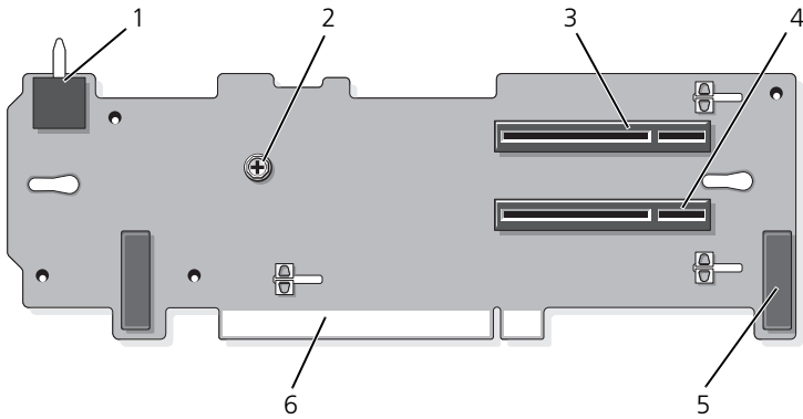
図 6-5. 標準 PCIe 拡張カードライザー 2 のコンポーネント
