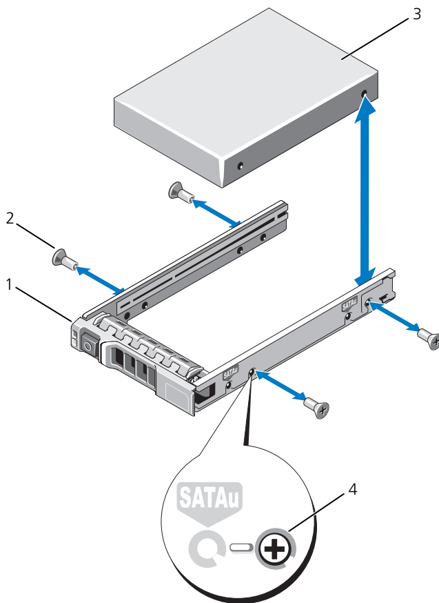
図 3-7. ハードディスクドライブのドライブキャリアへの取り付け
