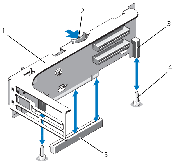
図 3-24. 拡張カードライザー 2 の取り外しと取り付け
