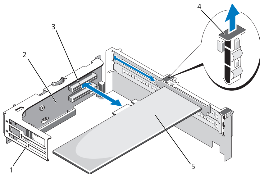
図 3-22. 拡張カードの取り外しと取り付け
