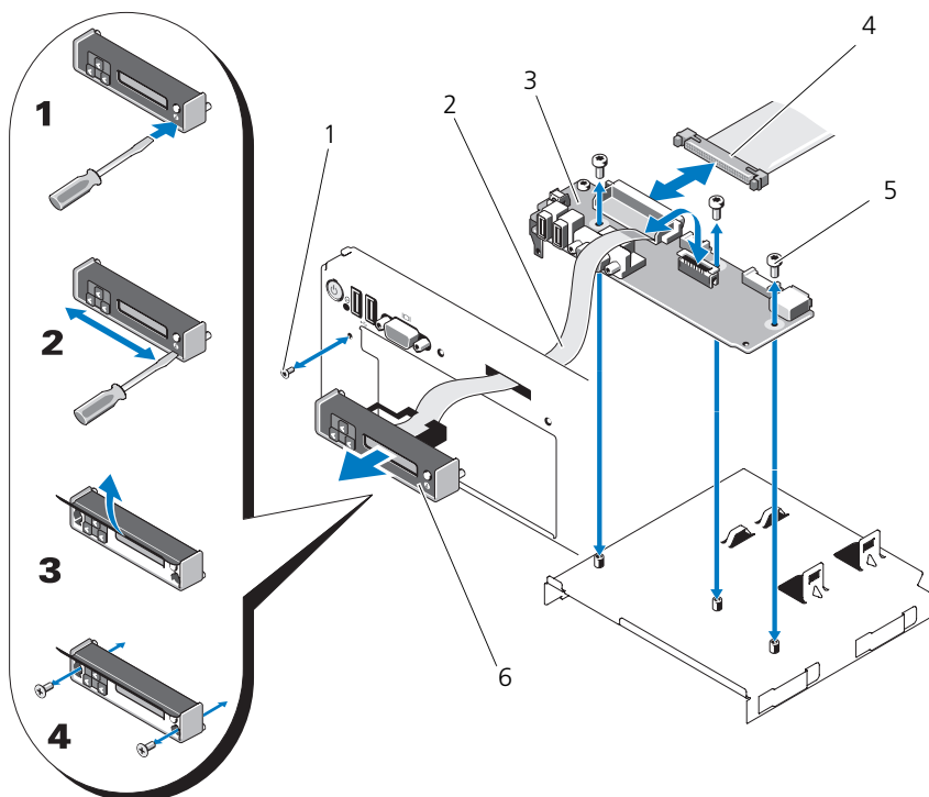
図 3-32. コントロールパネルの取り外しと取り付け
