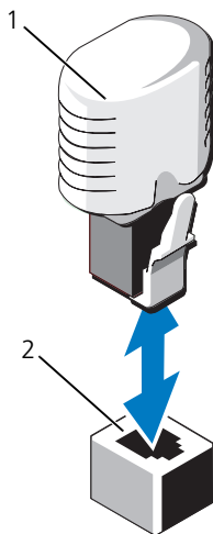
図 3-12. NIC ハードウェアキーの取り外しと取り付け
