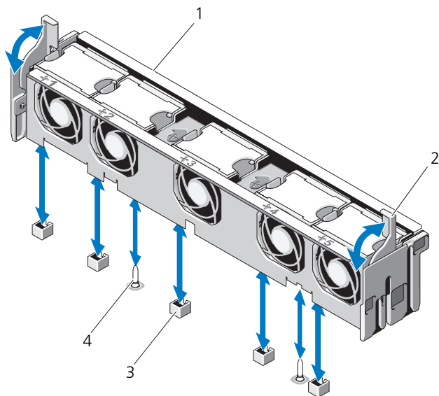
図 3-15. プロセッサファンブラケットの取り外しと取り付け
