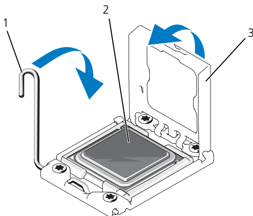
図 3-30. プロセッサシールドを閉じる
