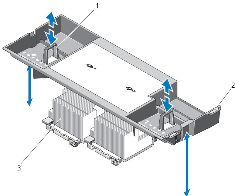
図 3-13. エアフローカバーの取り外しと取り付け
