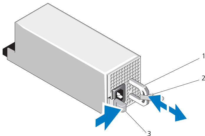
図 3-8. 電源装置の取り外しと取り付け
