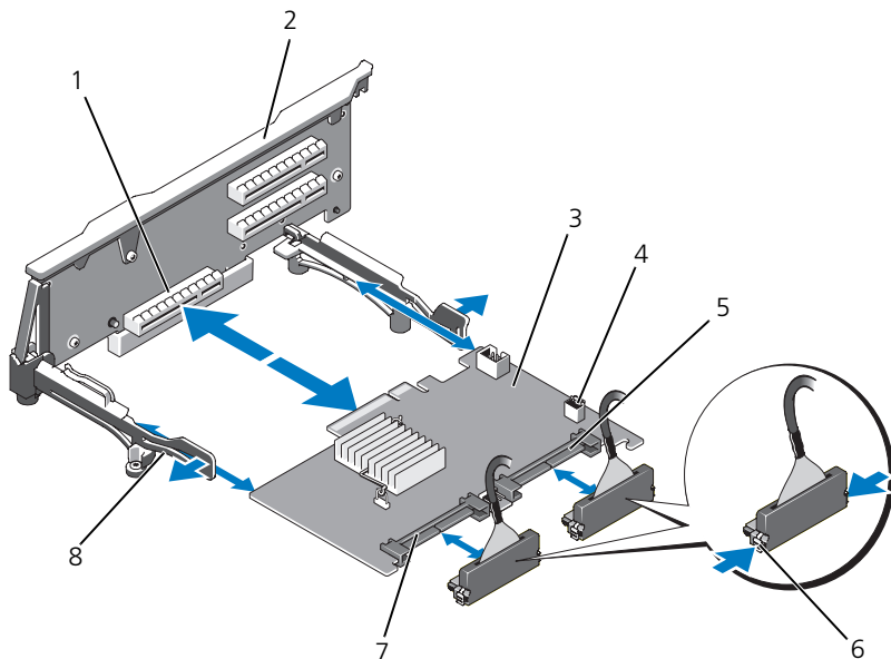
図 3-18. ストレージコントローラカードの取り付け
