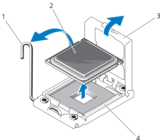
図 3-28. プロセッサの取り外し
