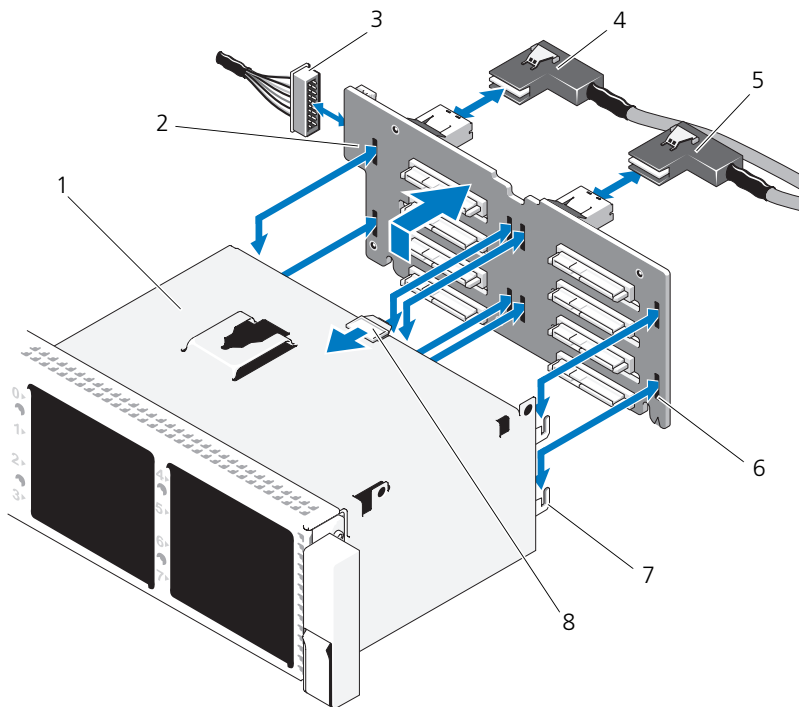
図 3-33. SAS バックプレーンの取り外しと取り付け
